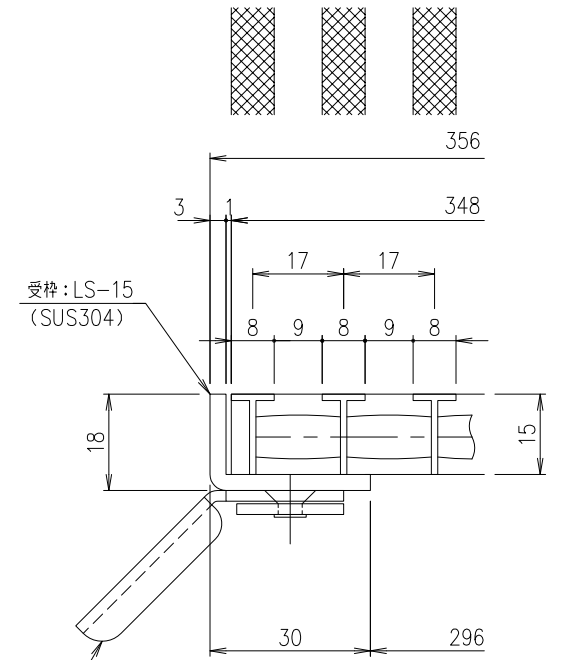
アンカー (SEHC) @500 受枠断面・メインバーピッチ詳細図 S=1/1
