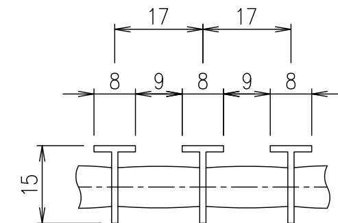
メンバーピッチ詳細図 S=1/1
