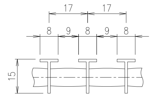
メインバーピッチ詳細図 S=1/1
