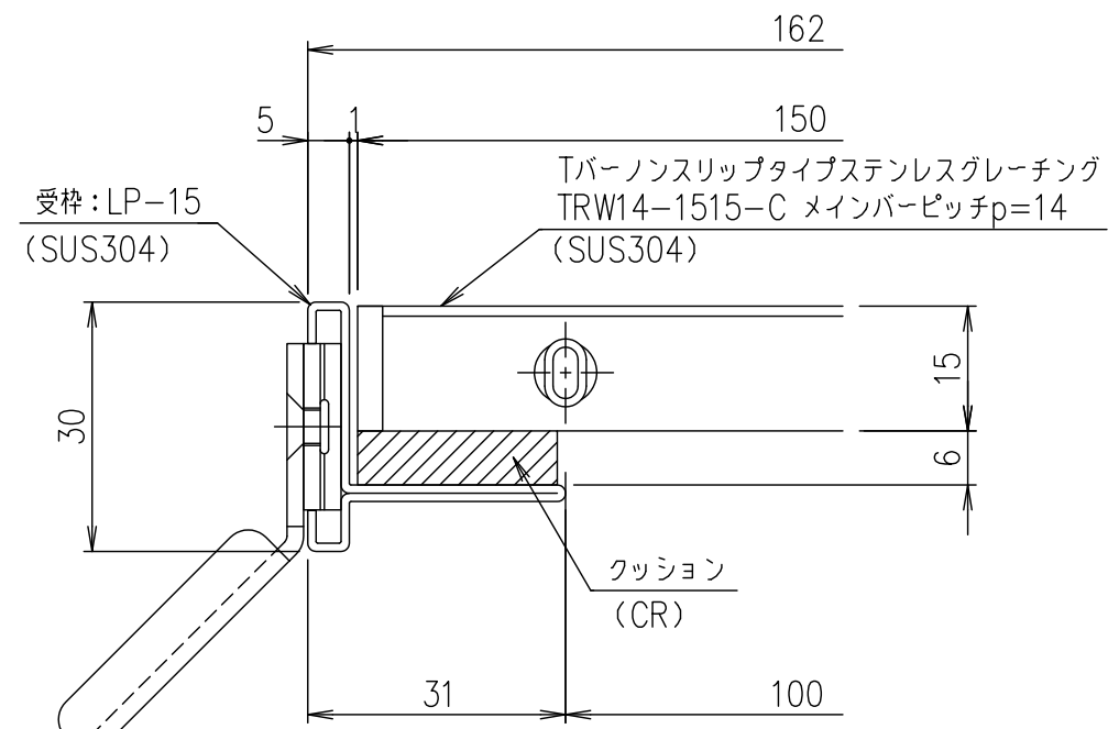
受枠断面詳細図 S=1/1
