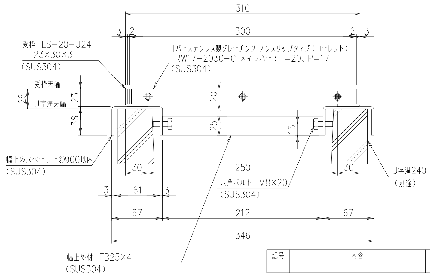
断面詳細図 S=1/3
