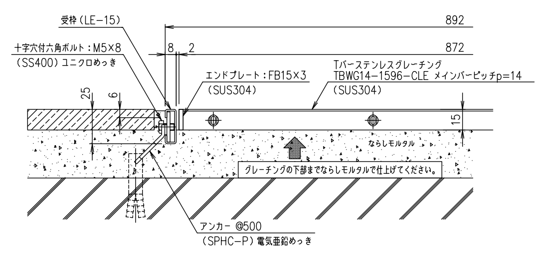
断面詳細図 S=1/2
