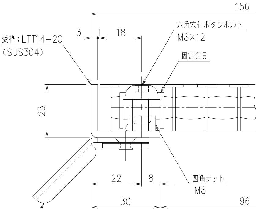
受枠断面詳細図 S=1/1
