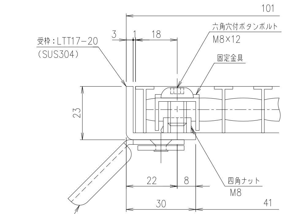
受枠断面詳細図 S=1/1
