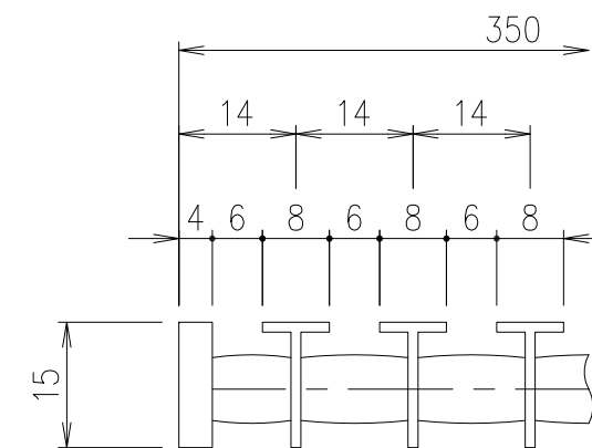
メインバーピッチ詳細
