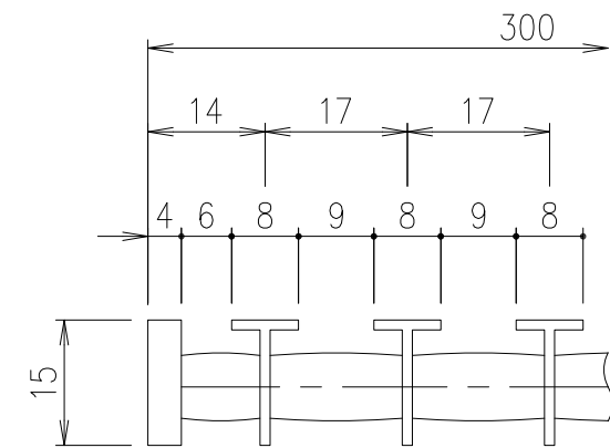
メインバーピッチ詳細
