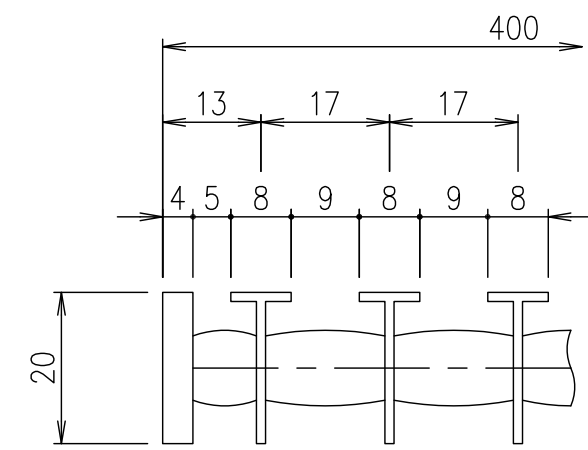
メインバーピッチ詳細
