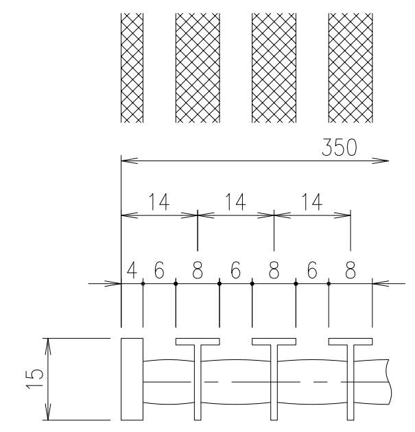
メインバーピッチ詳細
