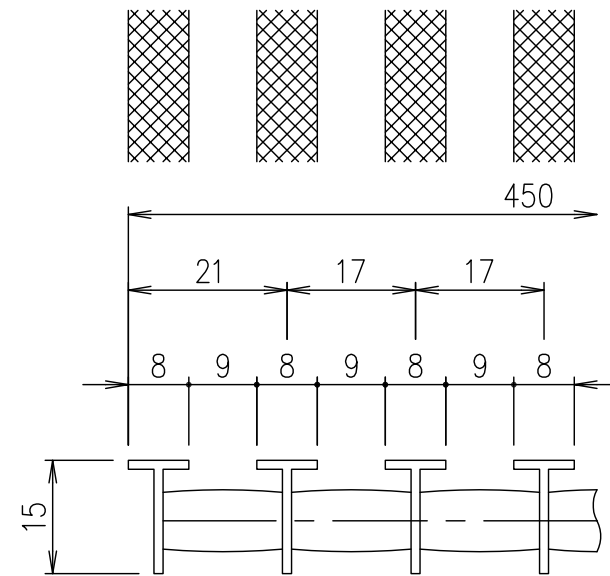
メインバーピッチ詳細
