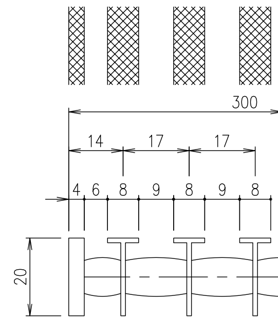
メインバーピッチ詳細
