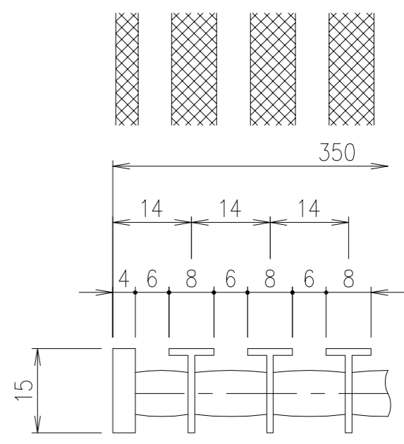
メインバーピッチ詳細
