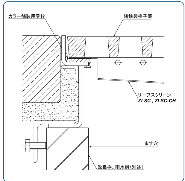
鋳鉄製格子蓋 カラー舗装用受枠
