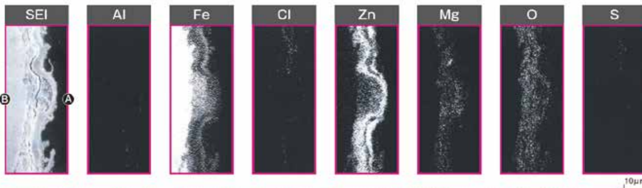
屋外暴露試験後の切断端面部断面状態(暴露18ヶ月後) (板厚: 2.3mm、めっき付着量: 130/130 g/m²)
