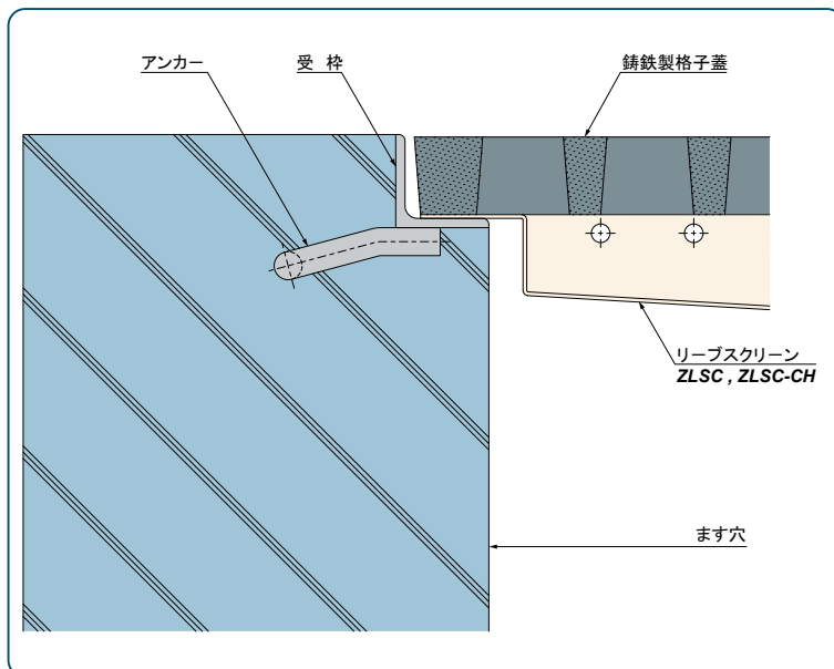
铸铁製格子蓋 一般用受枠
