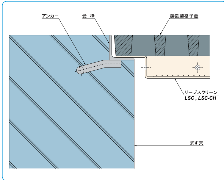
铸铁製格子蓋 一般用受枠
