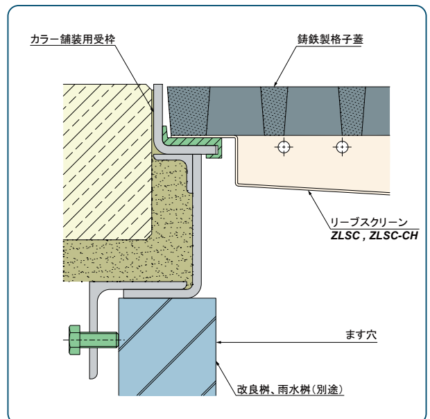
铸铁製格子蓋 カラー舗装用受枠
