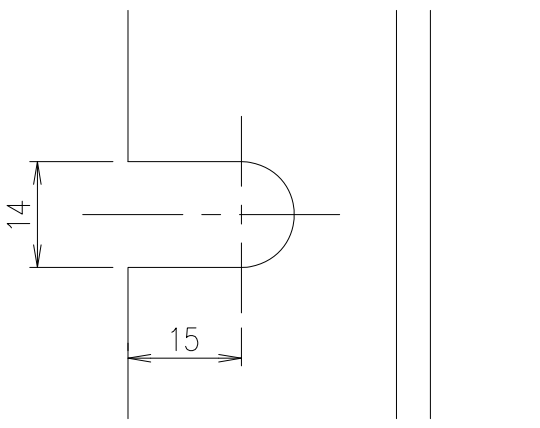
切欠き部 A-A 断面詳細図 S=1/1
