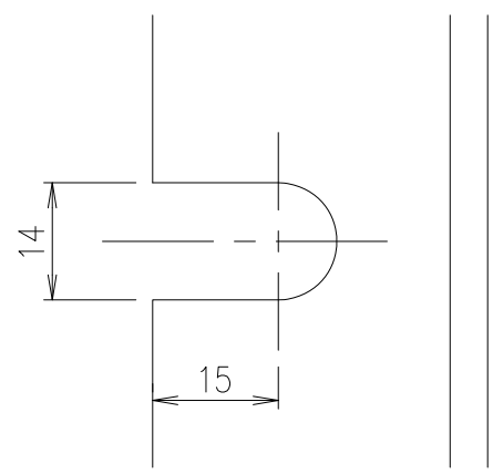
切欠き部 A-A 断面詳細図 S=1/1
