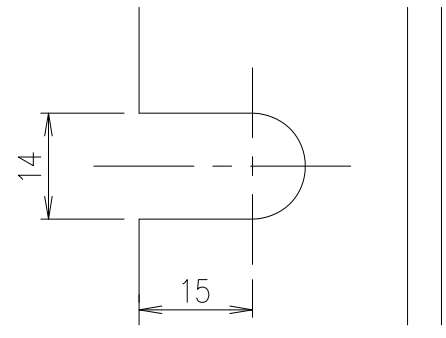
切欠き部 A-A 断面詳細図 S=1/1
