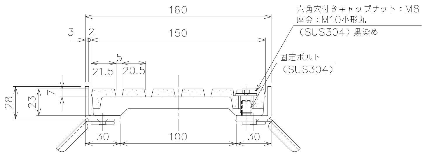
詳細図 S=1/2
