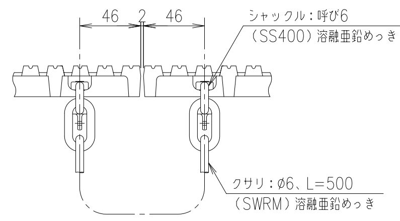
クサリ・シャクル取付け方法 S=1/3
