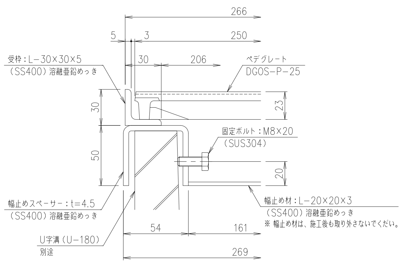
受枠 断面詳細図 S=1/2
