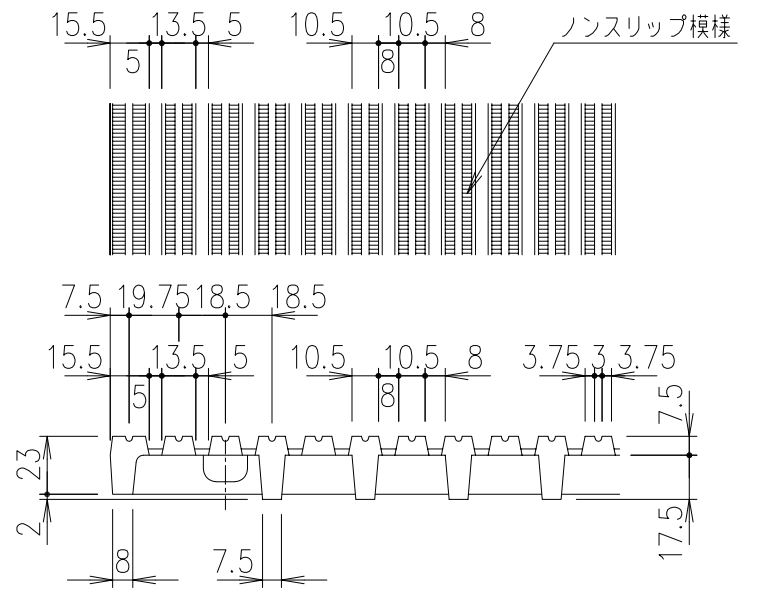
平面・断面ノンスリップ詳細図 S=1/3
