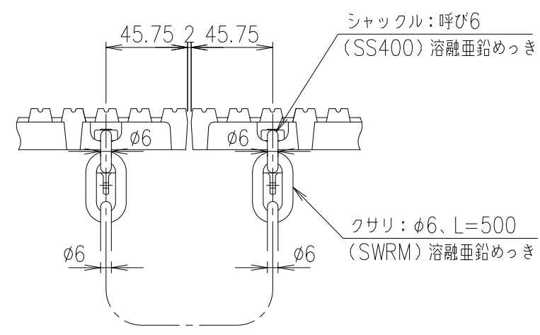
クサリ・シャクル取付け方法 S=1/3
