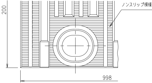
A 部 詳細図 S=1/1
