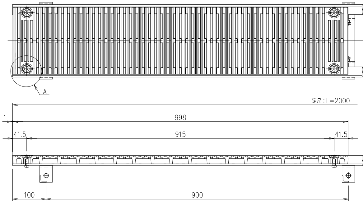
製品図 S=1/5
