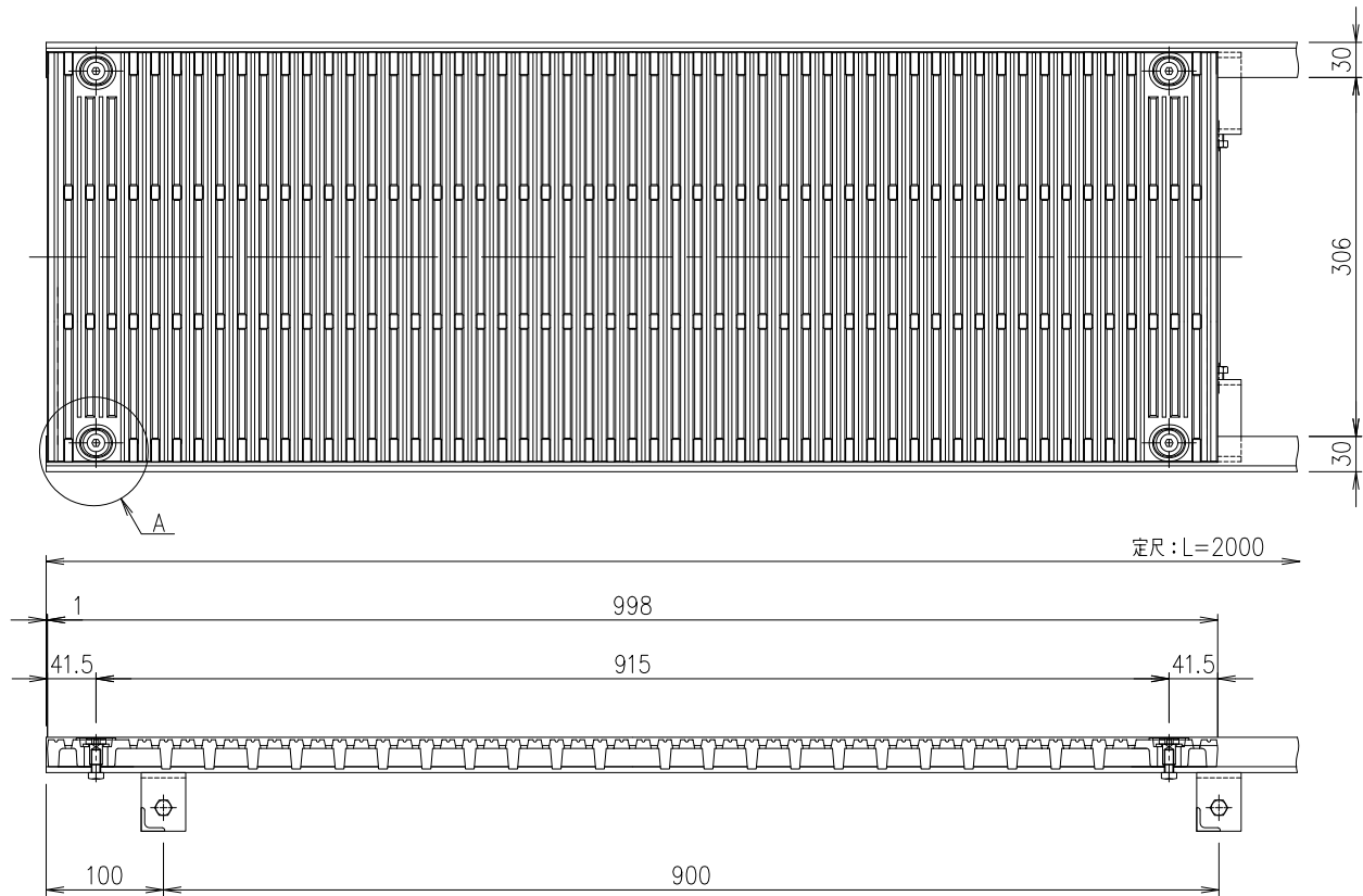
製品図 S=1/5
