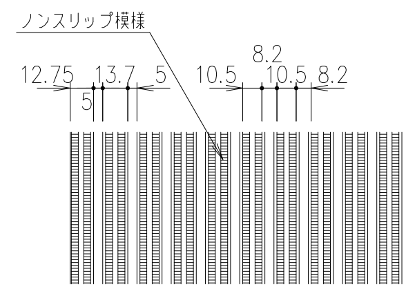
部分詳細 S=1/3
