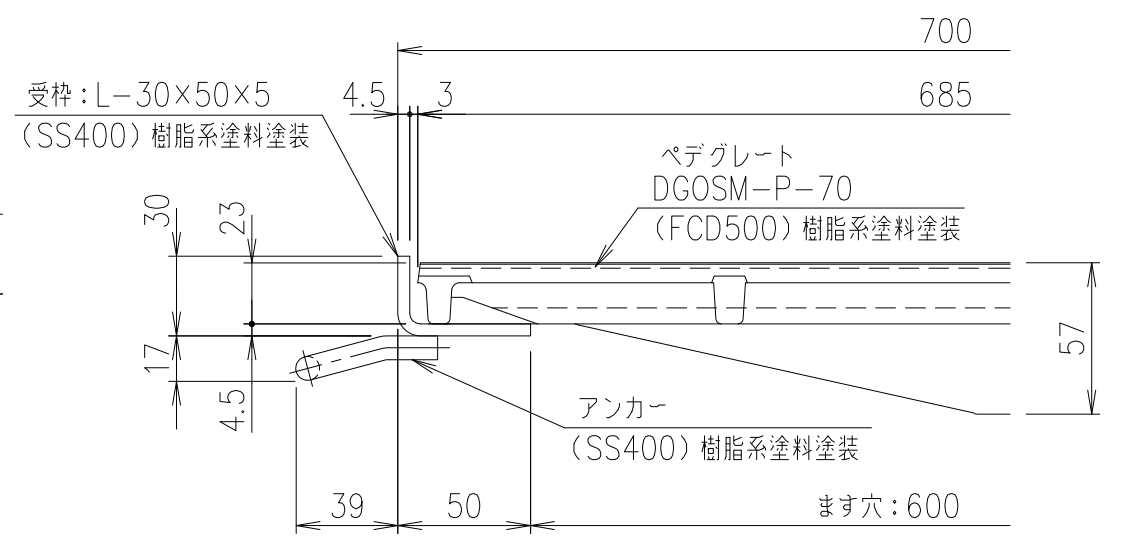
部分詳細 S=1/3
