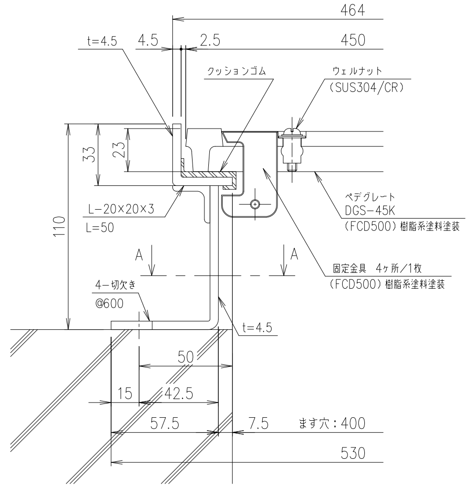
DGS-45K 断面詳細図 S=1/2
