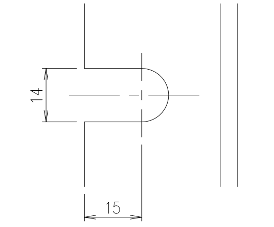
切欠き部 A-A 断面詳細図 S=1/1
