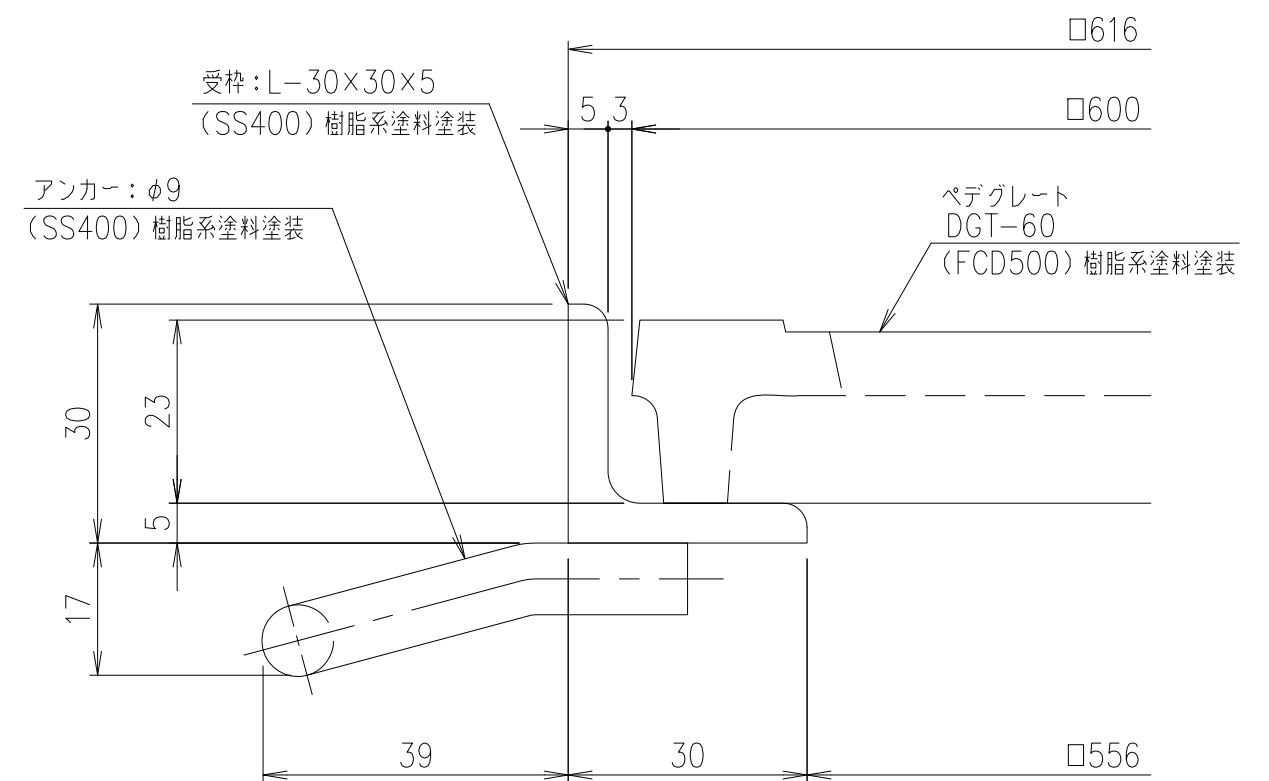
部分詳細
