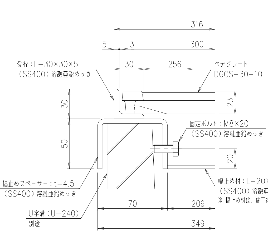
受枠 断面詳細図 S=1/2
