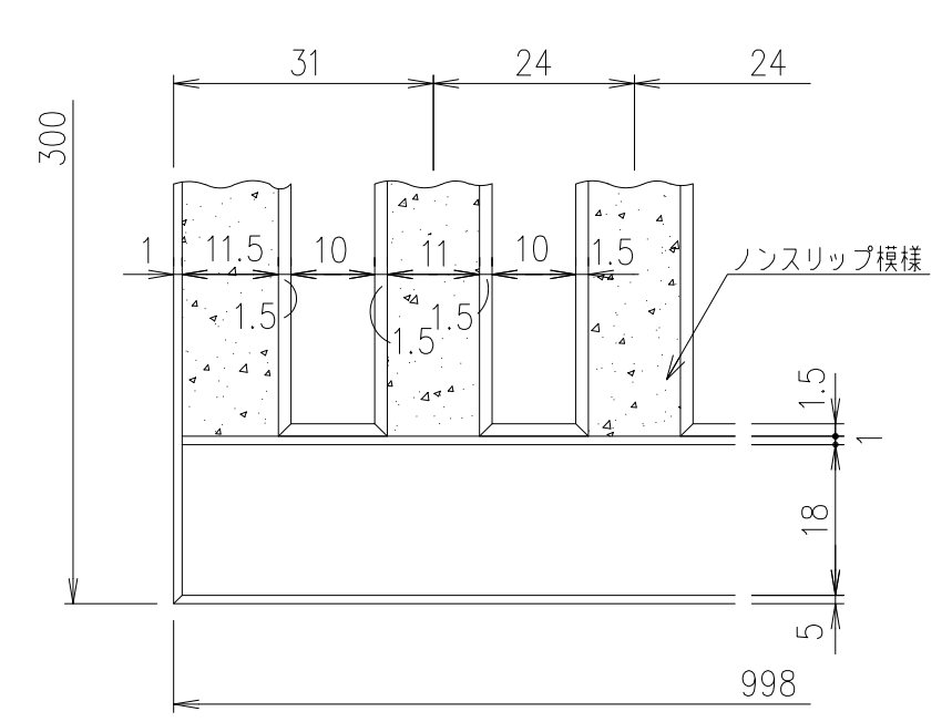
A部詳細
