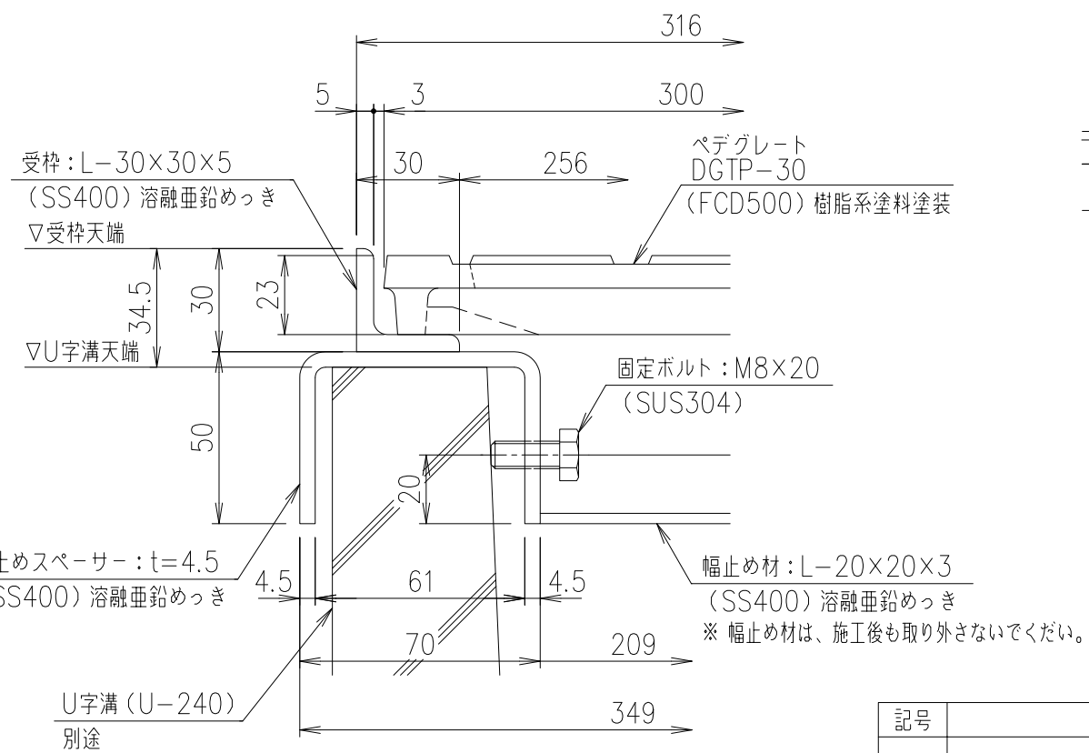
部分詳細図 S=1/2
