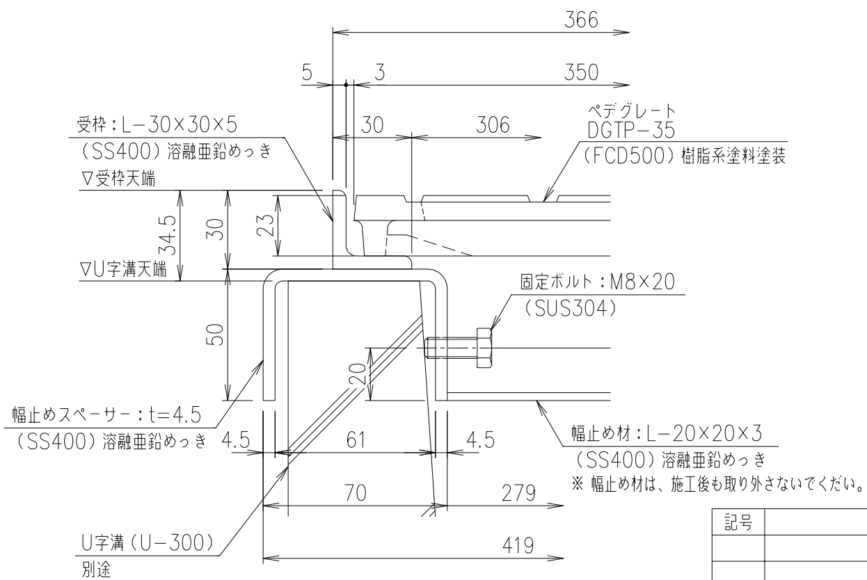
部分詳細図 S=1/2
