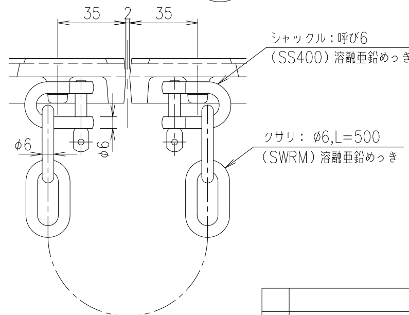
連結クサリ取付図 S=1/2
