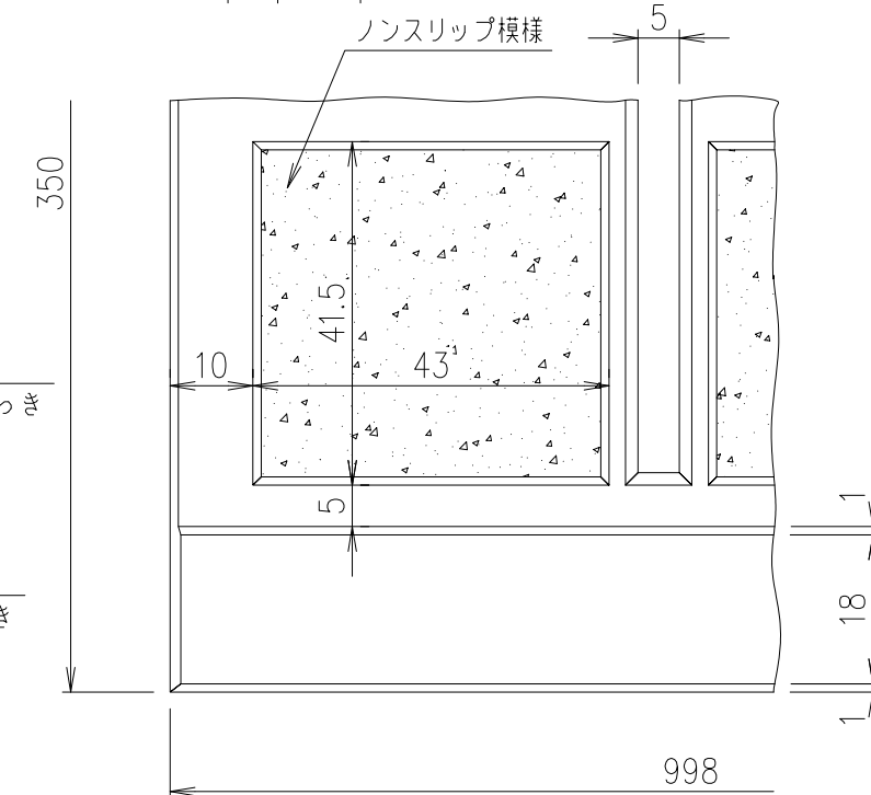
A部詳細
