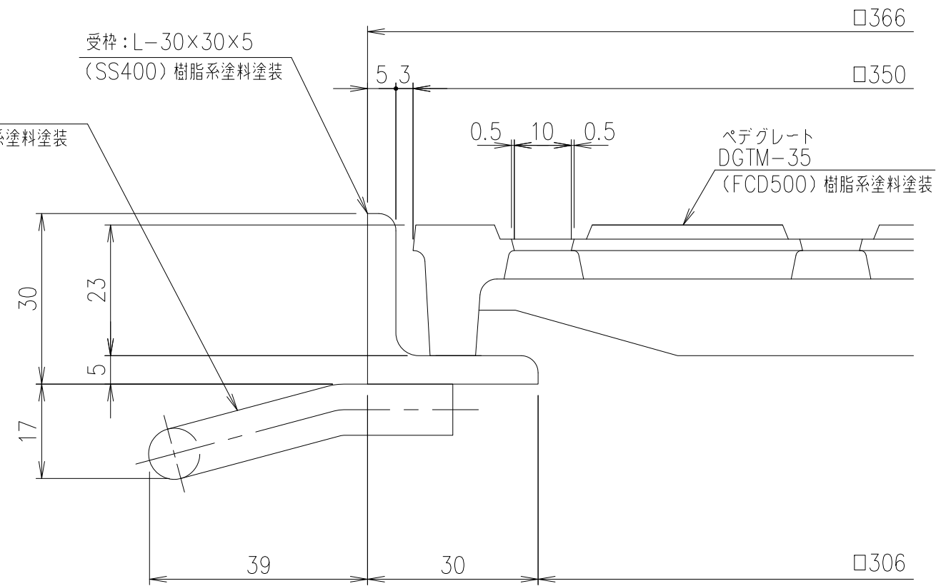
部分詳細
