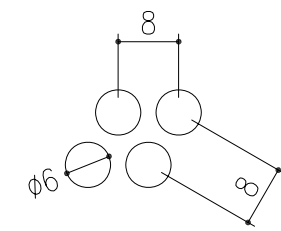
パンチング穴詳細図 S=1/1
