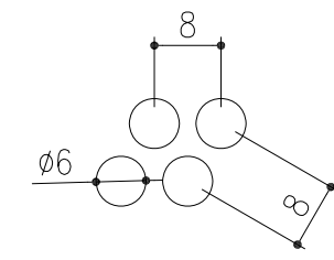
パンチング穴詳細図 S=1/1
