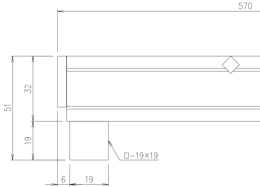
A部詳細図 S=1/1
