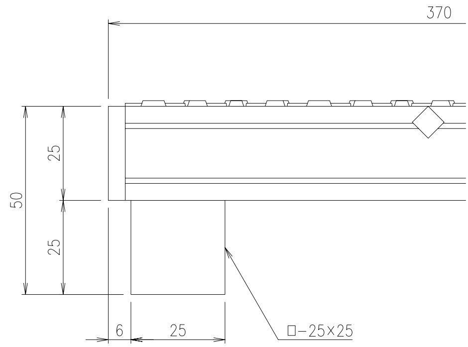
A部詳細図 S=1/1
