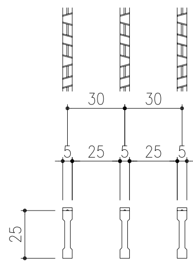
メインバーピッチ詳細図 S=1/2
