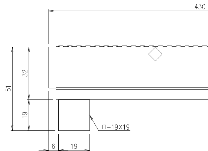
A部詳細図 S=1/1
