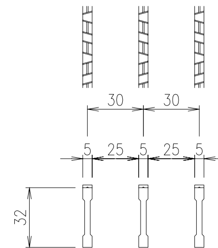
メンバーピッチ詳細図 S=1/2
