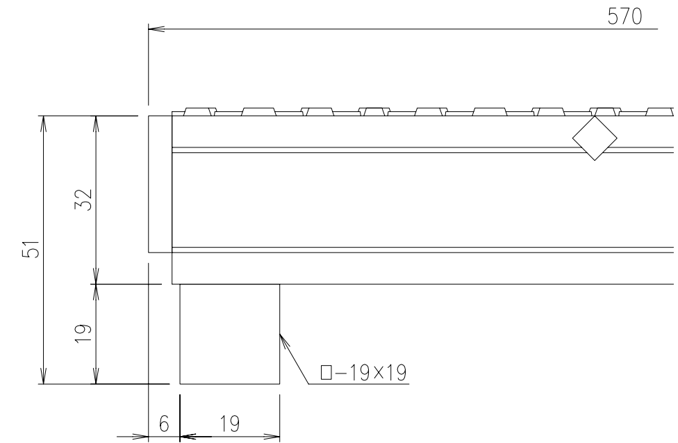
A部詳細図 S=1/1
