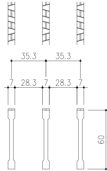
メンバー詳細図 S=1/2
