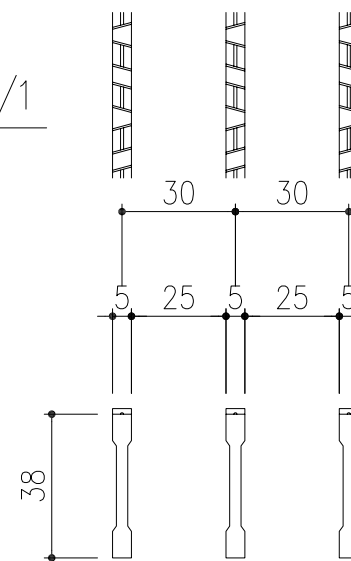
メンバーピッチ詳細図 S=1/2
