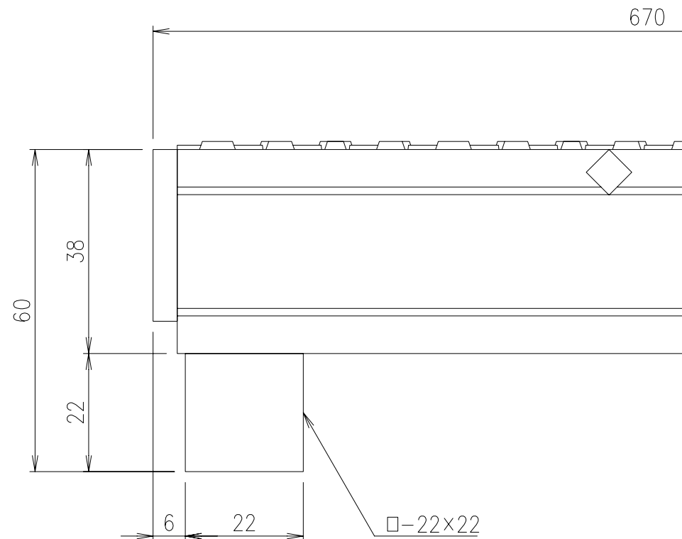
A部詳細図 S=1/1
