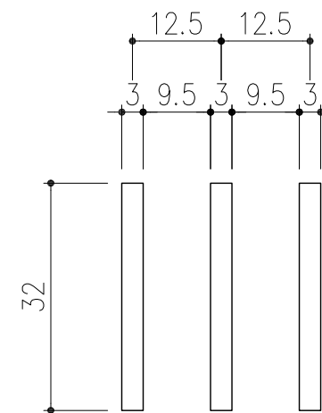
メインバーピッチ詳細図 S=1/1
