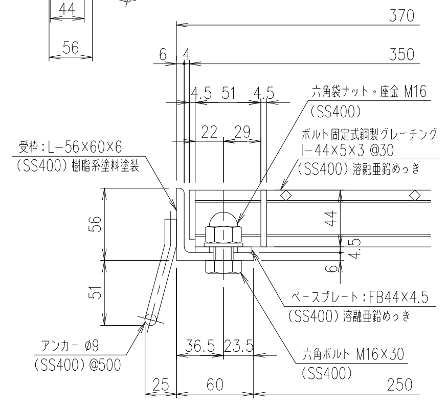
断面詳細図 S=1/3
