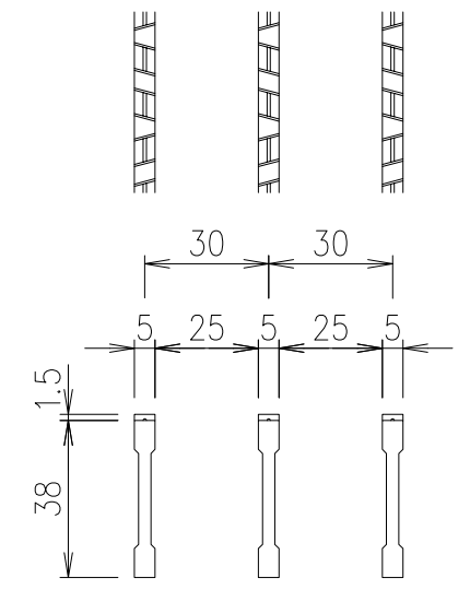
メインバー詳細図 S=1/2
