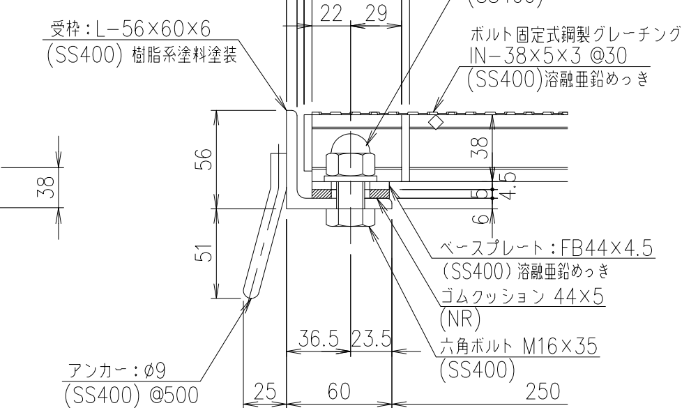
断面詳細図 S=1/3
