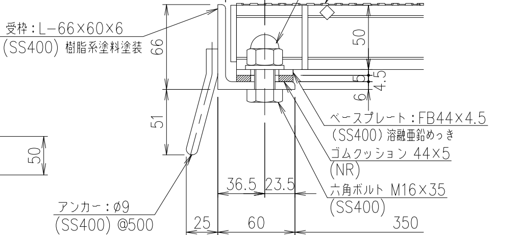
断面詳細図 S=1/3
