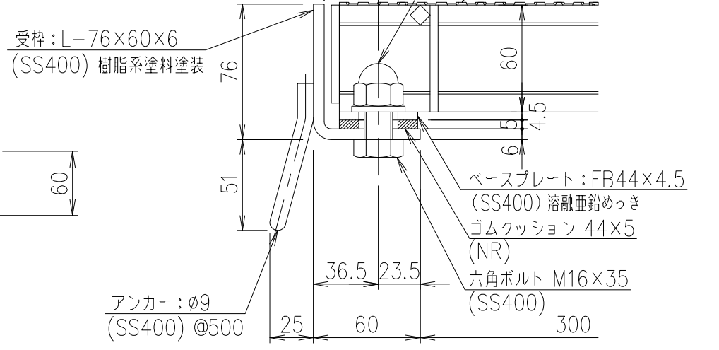
断面詳細図 S=1/3
