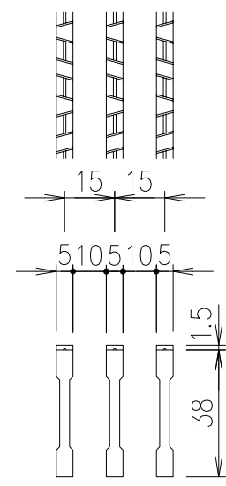
メインバー詳細図 S=1/2
