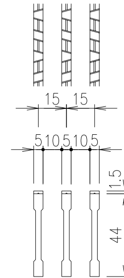
メンバー詳細図 S=1/2
